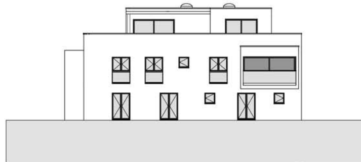
OSTFASSADE
